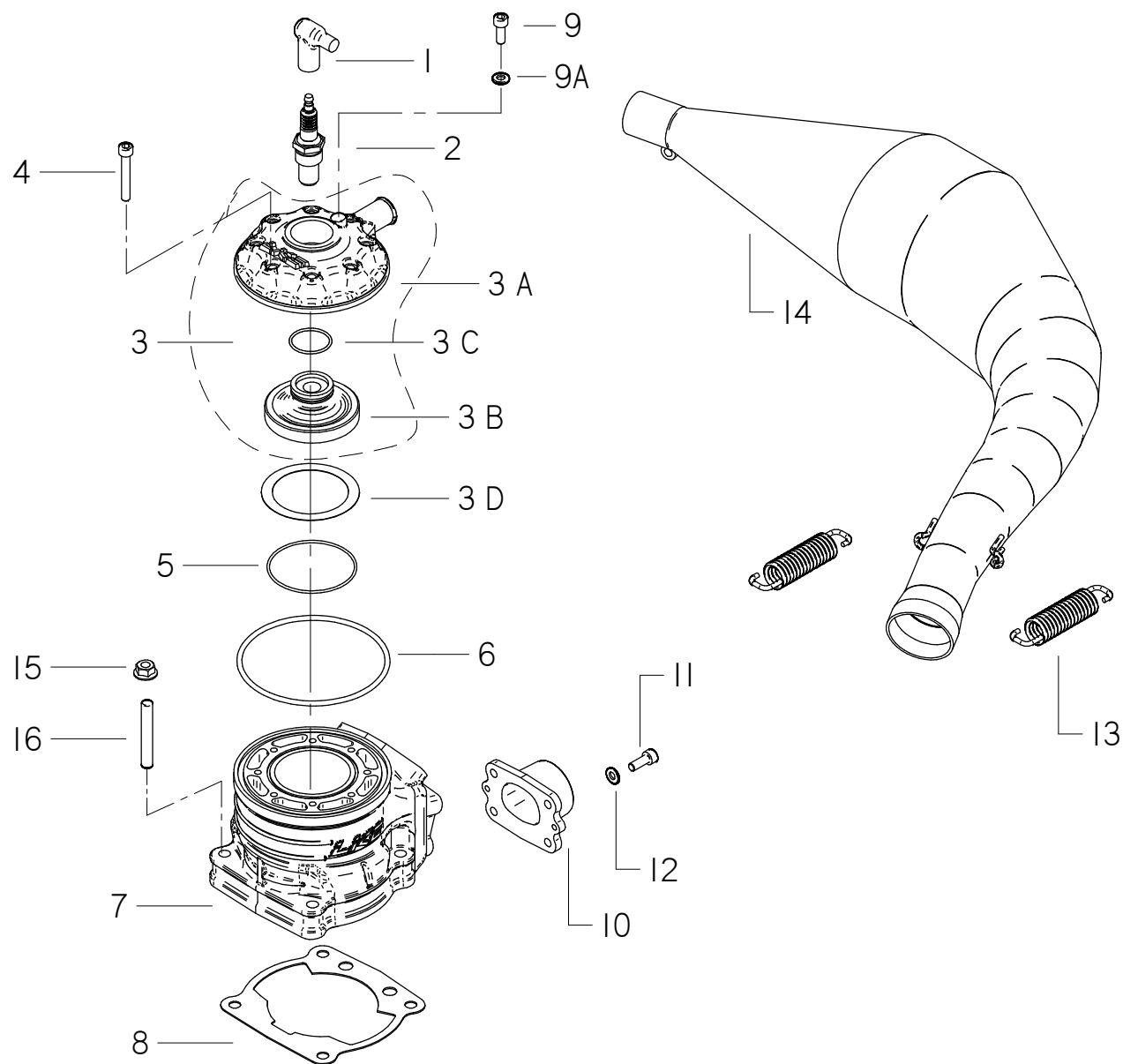
Gruppo cilindro motore LZI
