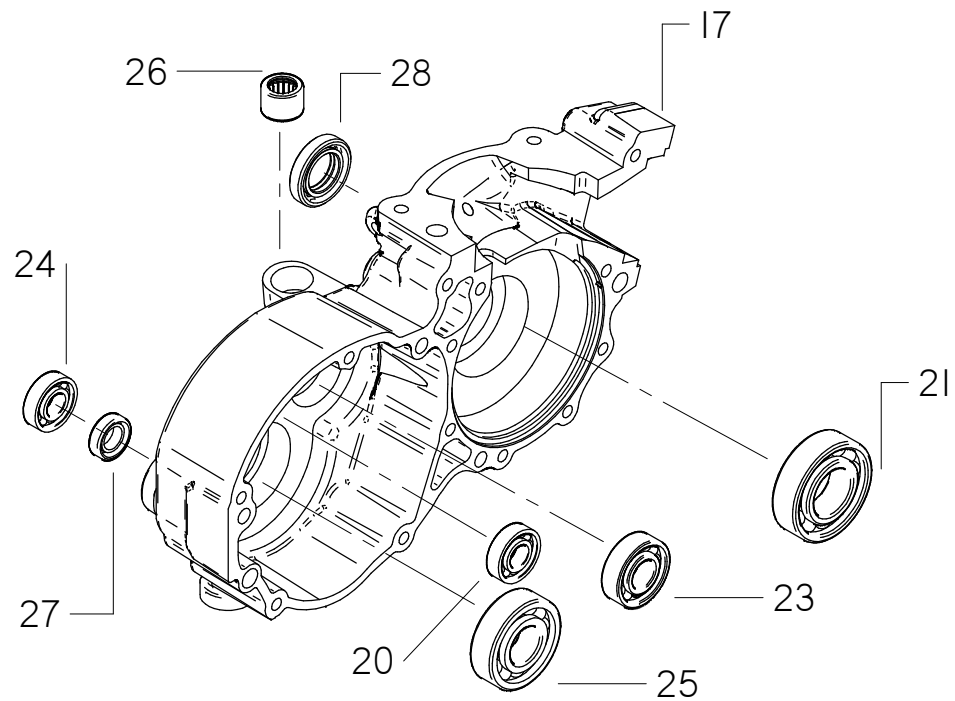
cuscinetti ed anelli di tenuta carter lato accensione motore LZI
