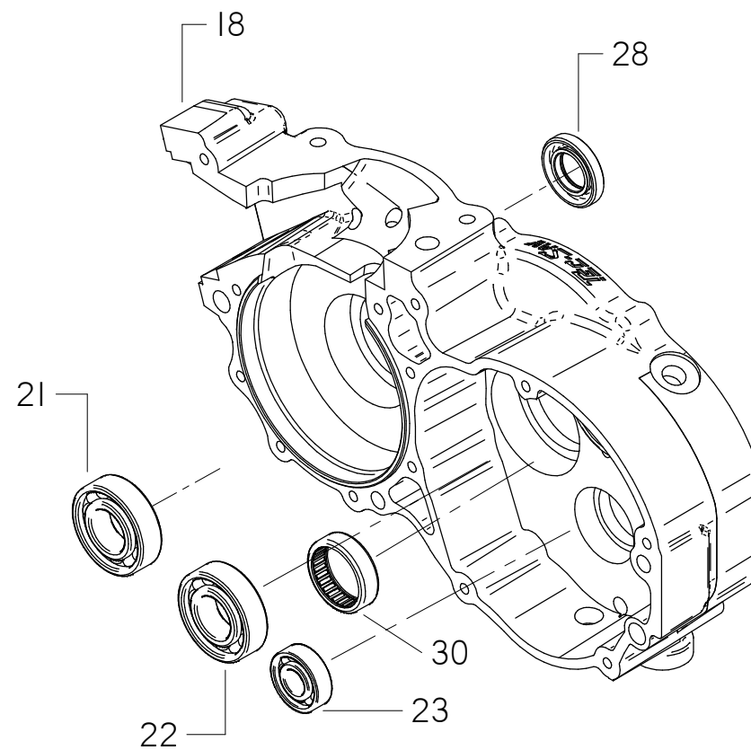
cuscinetti ed anelli di tenuta carter lato frizione motore LZI
