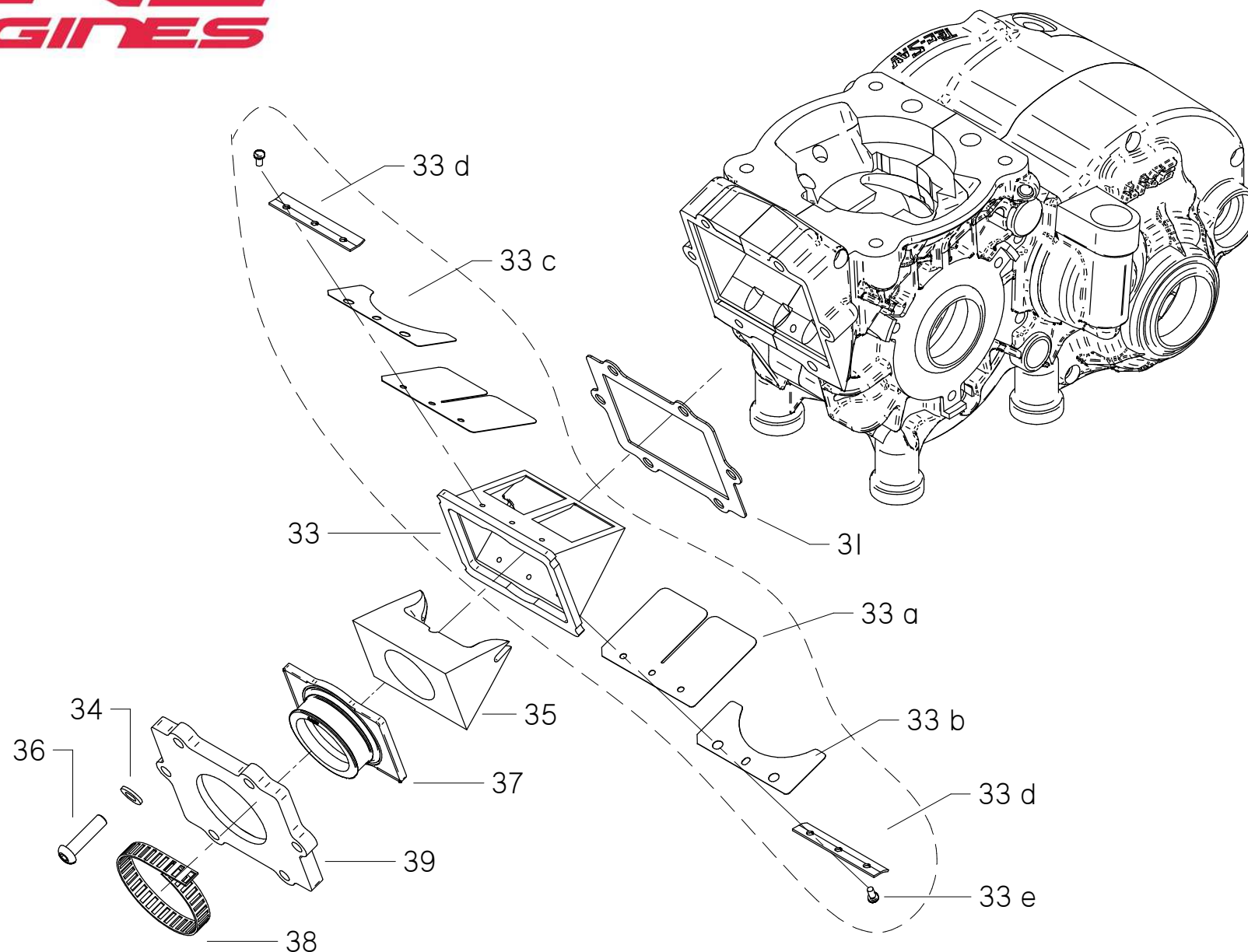
Gruppo pacco lamellare motore LZI
