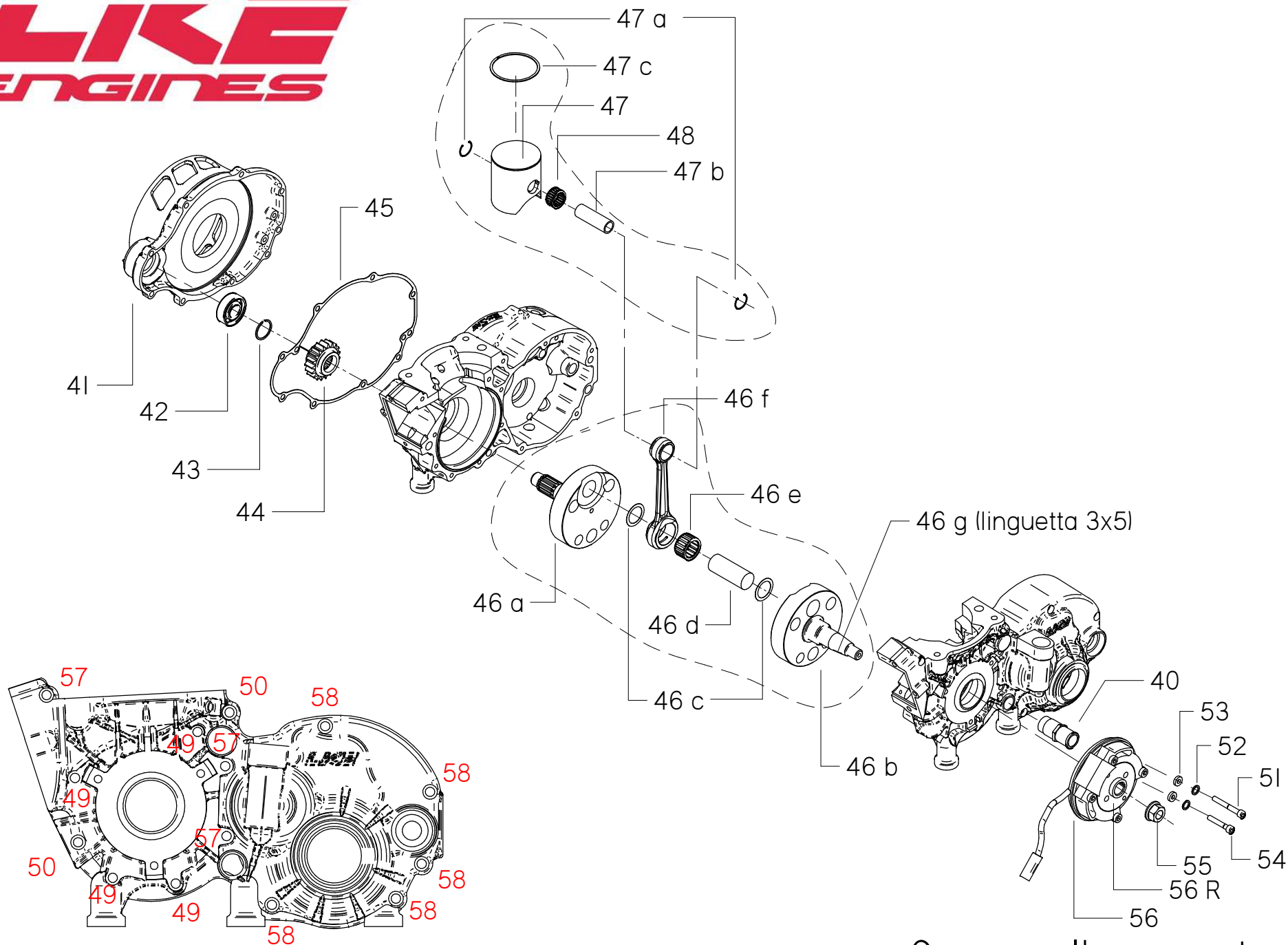
Gruppo albero motore LZI
